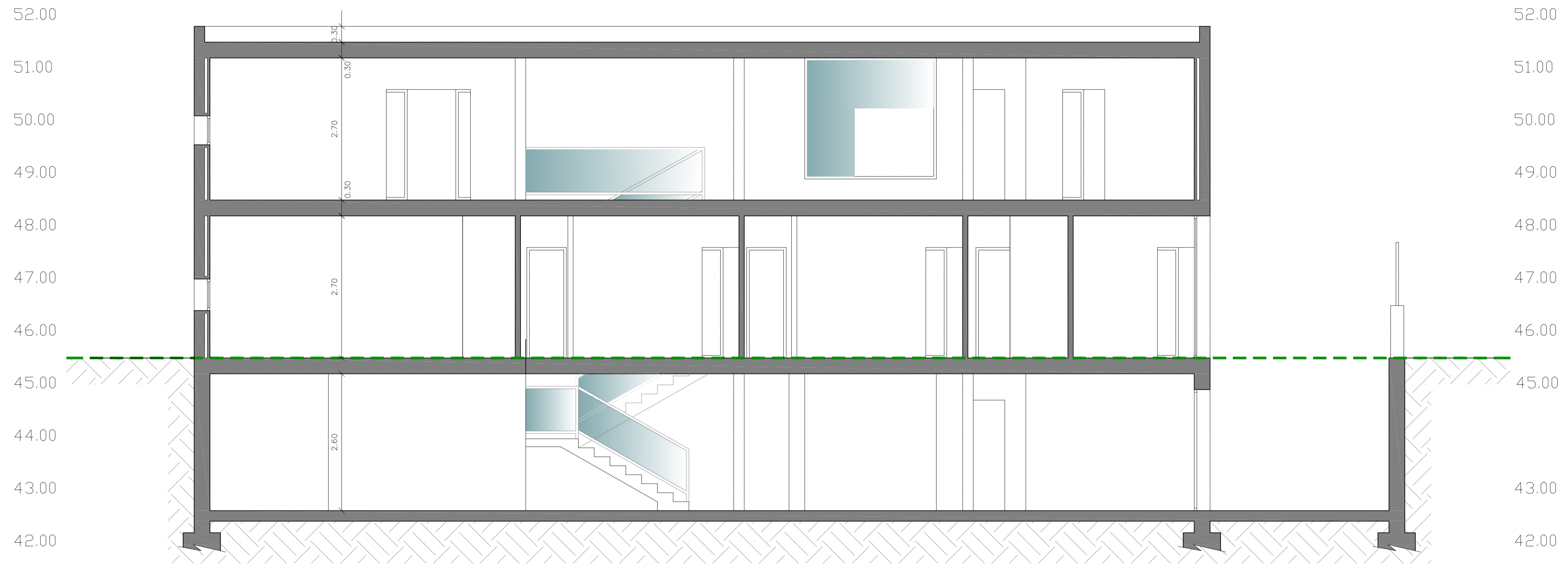
SECCION AA
