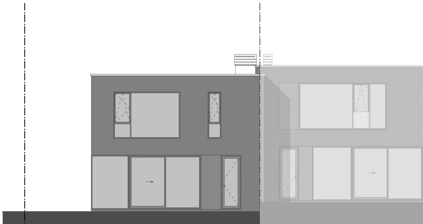
ACHTERGEVEL | 1:100
