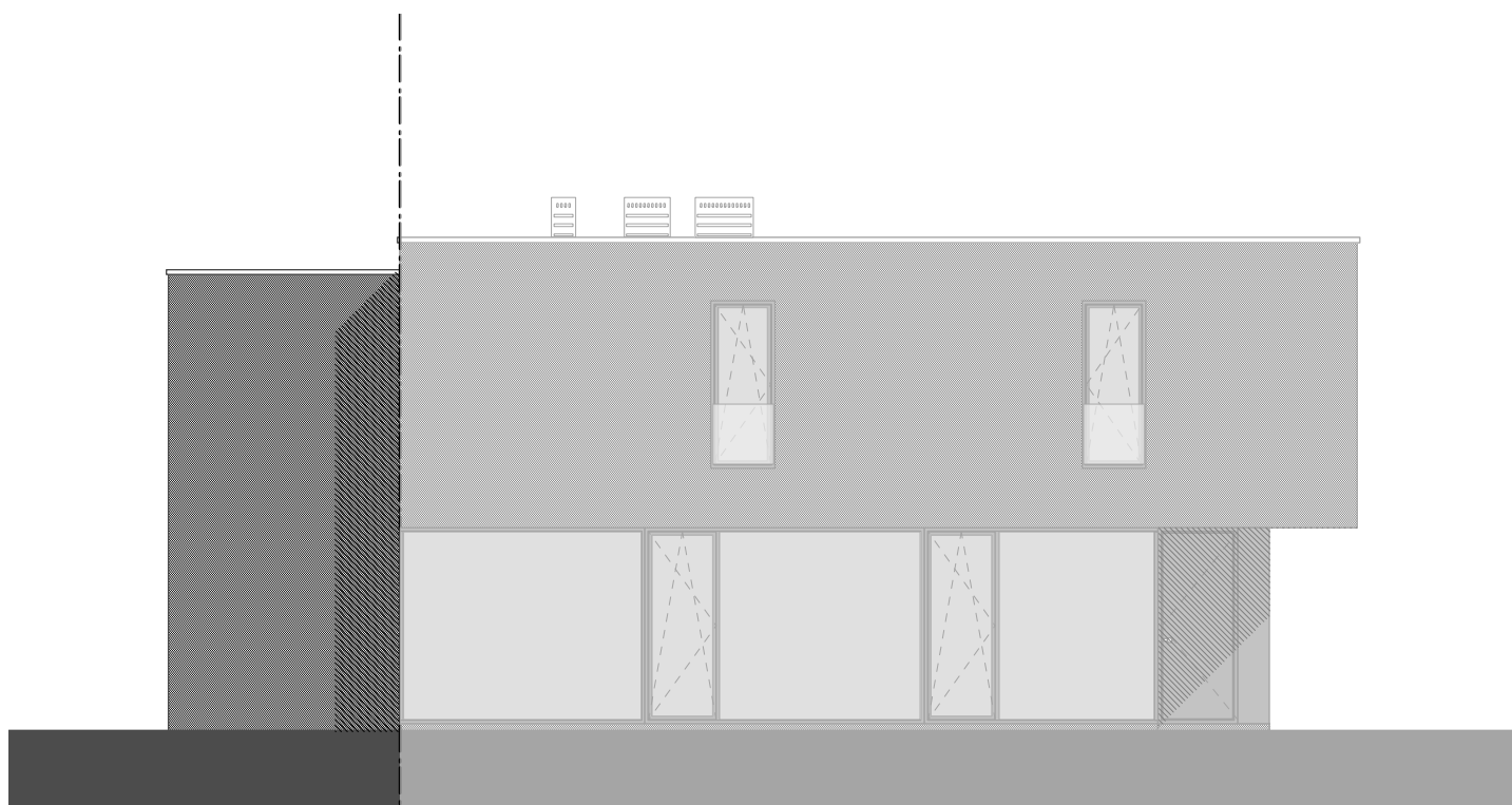
ZIJGEVEL LINKS | 1:100
